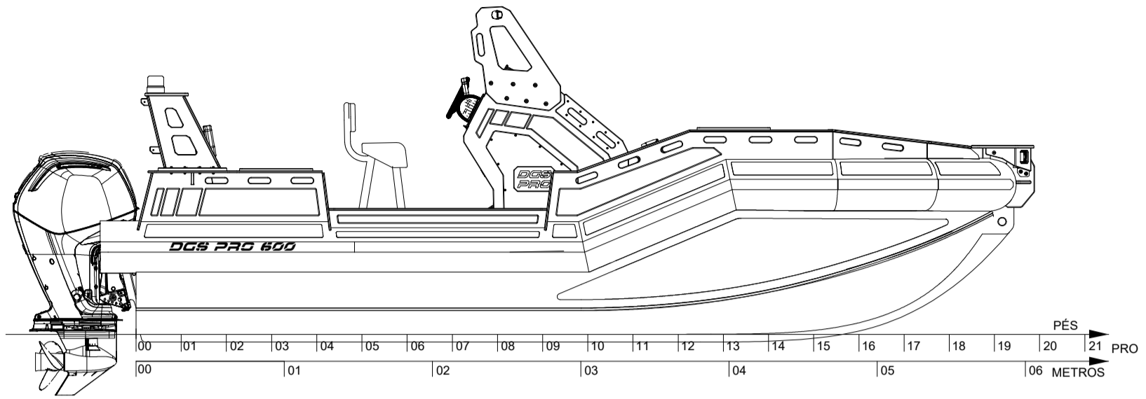
VISTA DE PERFIL EXTERNA
